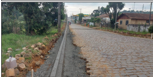
17 | Rua Cel. Tirburcio Cavalcante - meio fio em concreto
