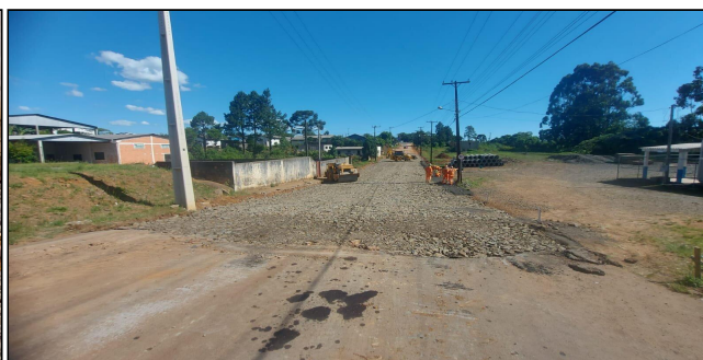
14 | Rua Cel. Tirburcio Cavalcante - Sub base em macadame
