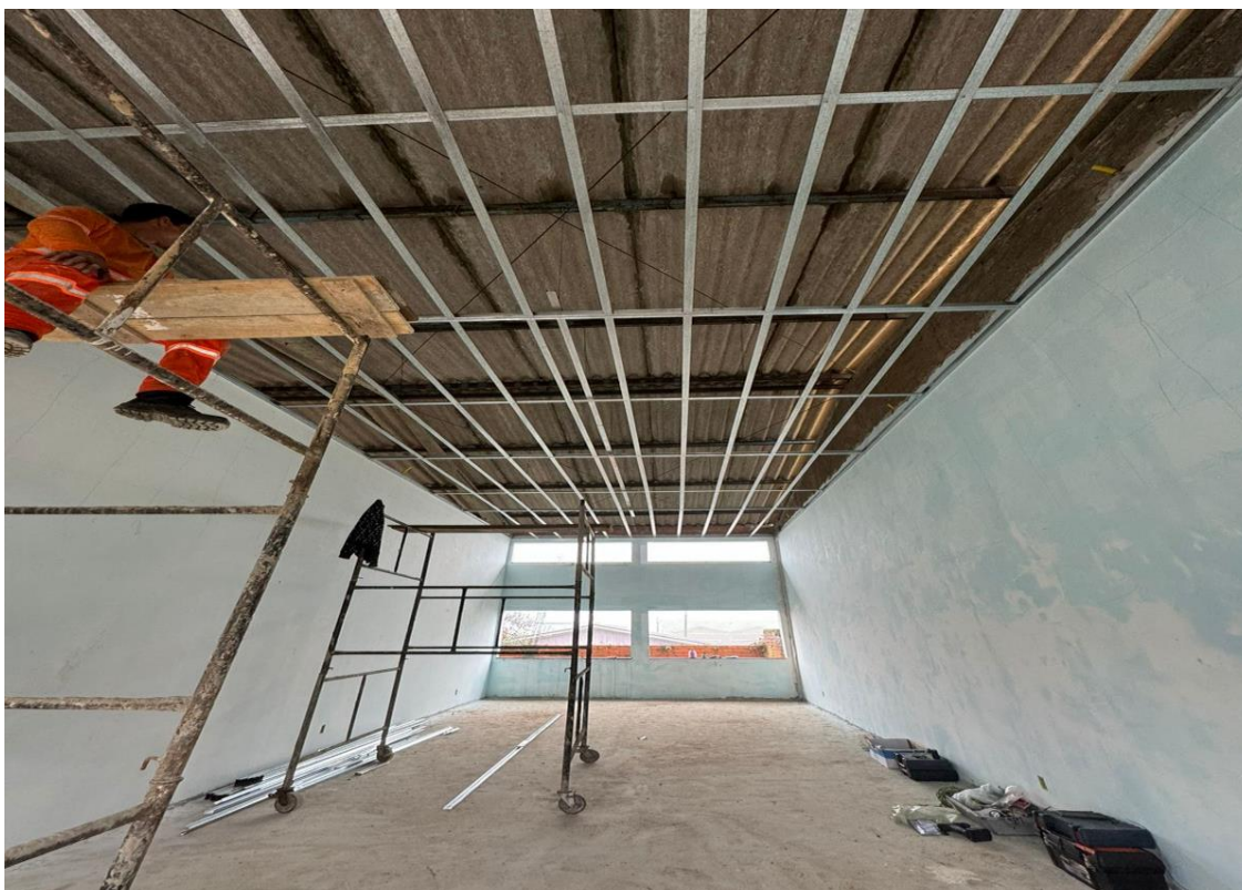
Imagem 09 – entarugamento em perfil metalico
