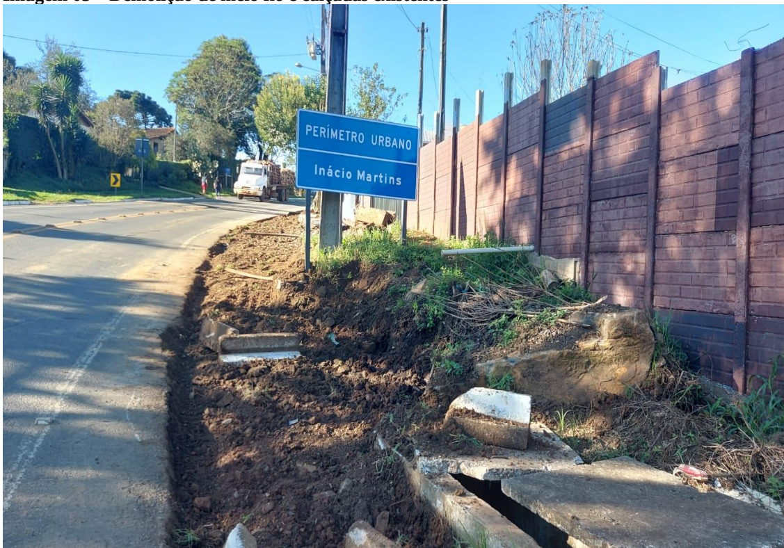
Imagem 03 – Demolição de meio fio e calçadas existentes
